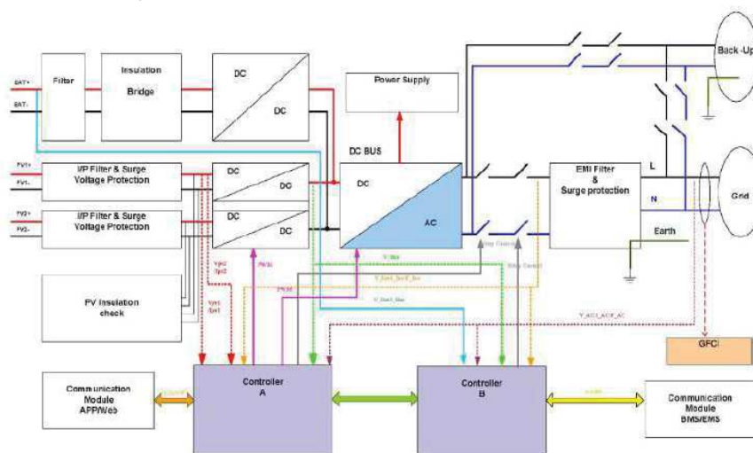
Gráfico 2 - Diagrama de bloques
